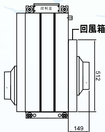
8"*1 單孔回風箱示意圖
