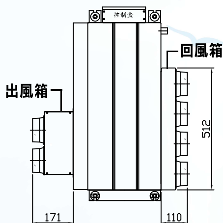
4"*4 四孔出回風箱示意圖
