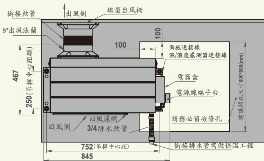
▲安裝重點及位置示意圖(MD-70LB)
