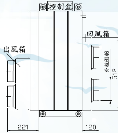
6"×2 雙孔出回風箱示意圖
