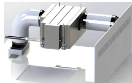
▲ 下回風 / 側出風
