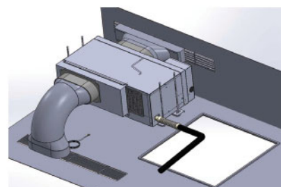
▲ 下側回風側邊出風
