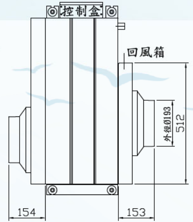
8"×1 單孔回風箱示意圖
