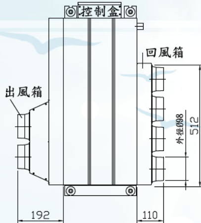
4"×4 四孔出回風箱示意圖
