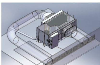
▲ 同側出回風
