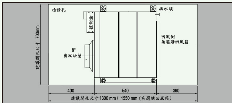
▲安裝尺寸參考(以MD-70LBA為例)
