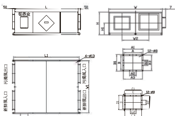
懸掛式 MHQ-D15~30TGTZ
