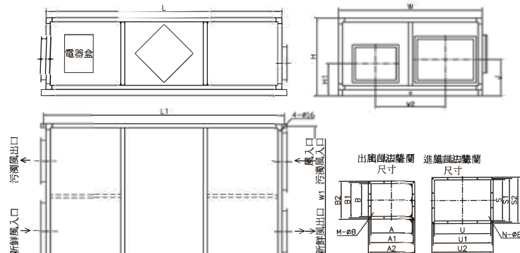
懸掛式 MHQ-D40~60TGT
