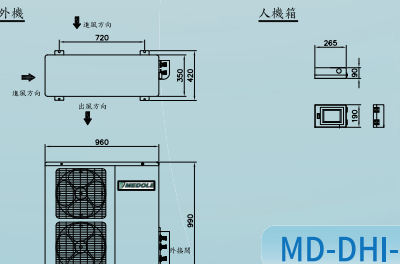
室外機
