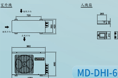
室外機
