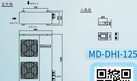
室外機
