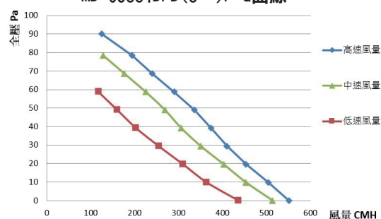
MD-65881DPD(8") P-Q曲線
